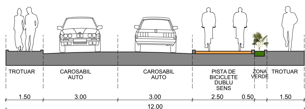
PROFIL DRUM PROPUIS 12.00 m prelungire str. Bartok Bela
